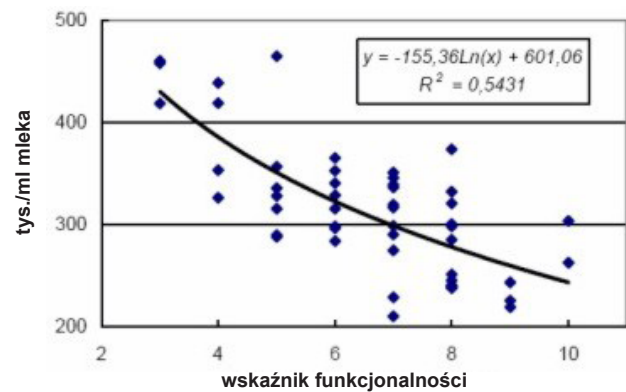
Rys. 3. Zależność między liczbą komórek somatycznych w mleku a wskaźnikiem funkcjonalności obory ( Wf ) obory ( r =-0,737 i R 2 =54,31%, standardowy błąd estymacji = 43,558)
