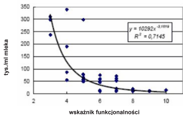
Rys. 4. Zależność między ilością drobnoustrojów w mleku a wskaźnikiem funkcjonalności obory ( Wf ) obory ( r =-0,845 i R 2 =71,45%, standardowy błąd estymacji = 52,017)
